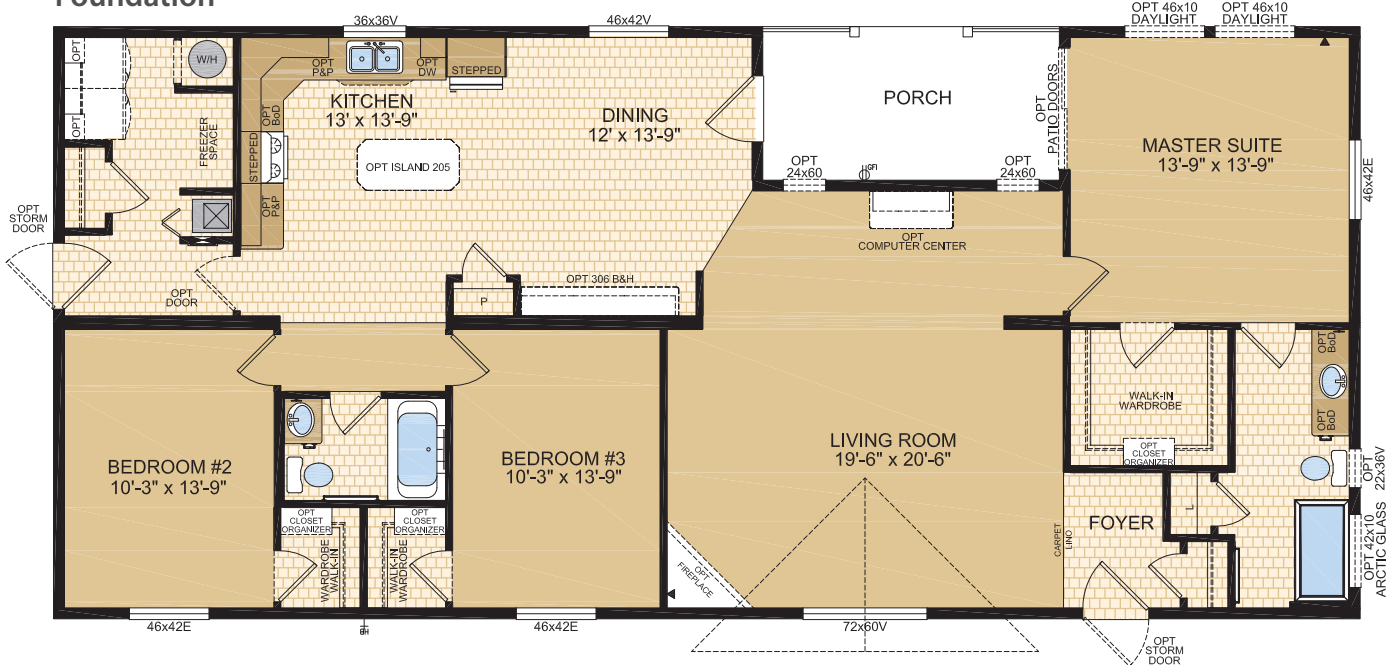
Optional Foundation
